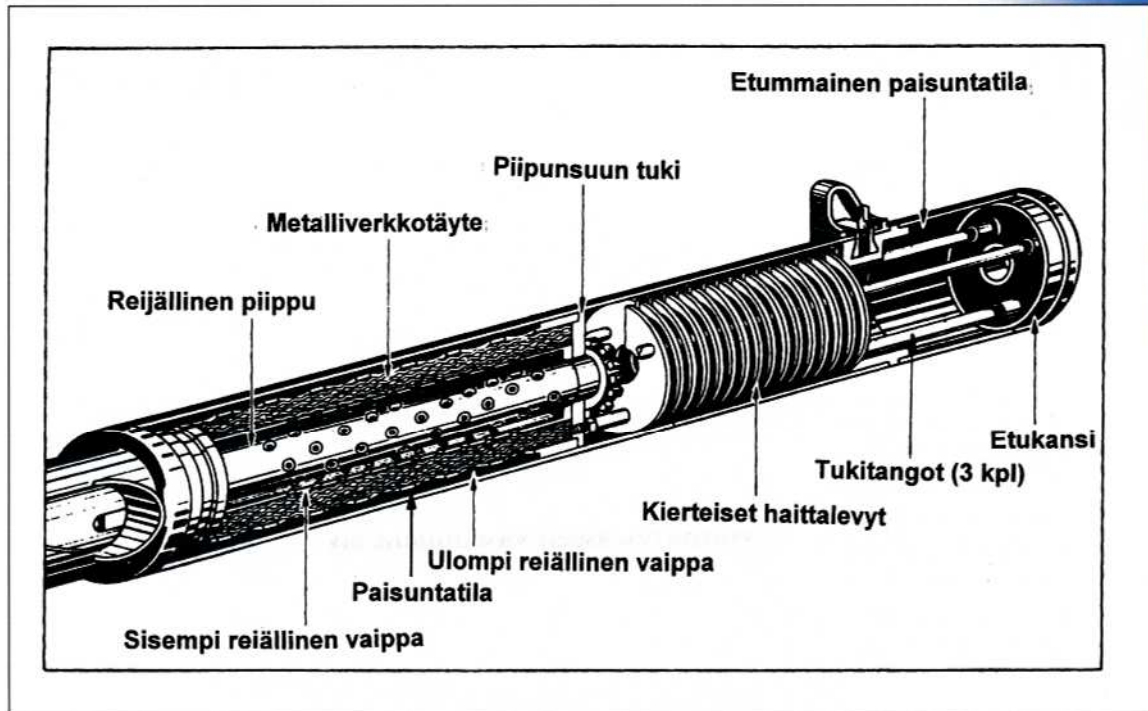
B. Kiintovaimentimen rakennepiirros
