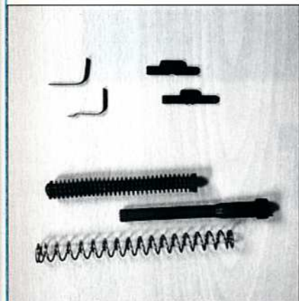
LMS-1141 laser-maalinosoitin korvaa GLOCK-pistoolin palautinjousen ja sen karan. Pistoolin alkuperäinen purkusalpa korvataan sivusuunnassa liikkuvaan. Uusi purkusalpa toimii käyttökytkimenä.
