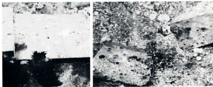
80 mm panssariteräs ennen ja jälkeen pohjamiinan räjäytyksen Sotinpuruolla.
