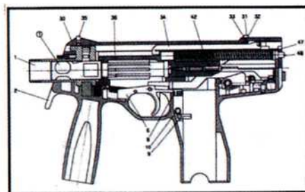
Halkileikkauspiirros mekaanisesta rakenteesta.
